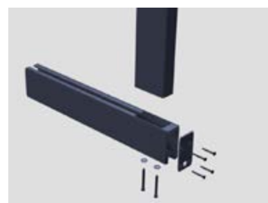
Tenons mortaises double cloison et vissage 2 points
