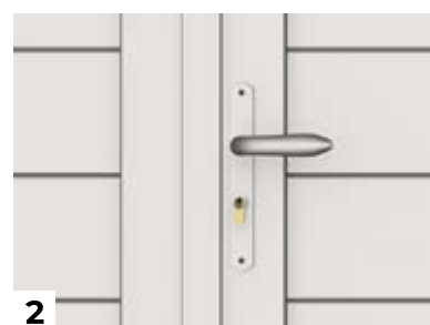
2 Poignée ronde avec plaque d'entrée laquée à la couleur du portail. Cylindre 30x30 mm Serrure encastrée 3 clés
