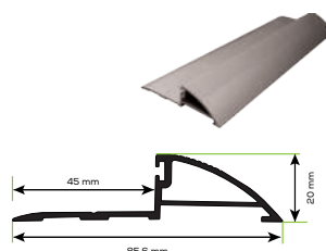
Seuil Alu
