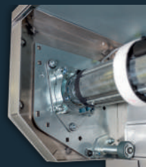
Joue acier sur silent-bloc Roulette souple anti-bruit
