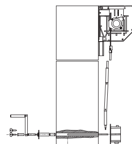
Manœuvre de secours Intérieure - Extérieure
